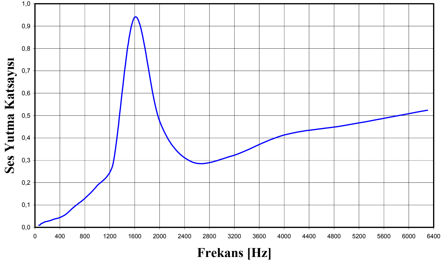
Şekil 6. “Polietilen sünger (kalınlık: 25 mm ) + Ağır bariyer (kalınlık: 4,6 mm)” malzemesinin ses yutma katsayısının frekansa bağlı olarak değişimi.
